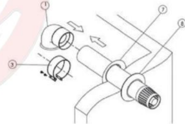
شکل ۱۲: خروجی دیواری دودکش دو جداره شکل ۱۳: نصب بخش های مجموعه دودکش هموستریک پکیج
