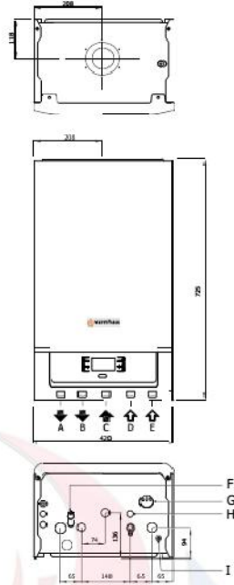
شکل ۷:بعاد و اتصالات لاپلاس پکیج
