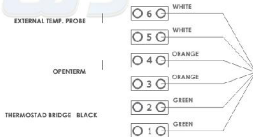
شکل ۲۱: اتصالات ترموستات اتاقی و سنسور دمای هوای خارجی پکیج
