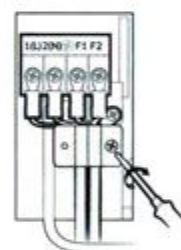
پیچ‌های مخصوص نگهدارنده‌های سیم را سفت کنید.
